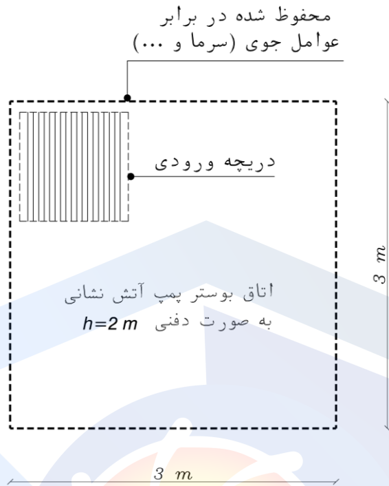
شکل پ-۶-۲- اتاق پمپ آتش‌نشانی (نمای پلان)
